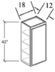
W1842
