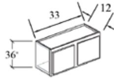
W3336
